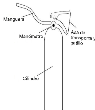
Imagen 6.4: Componentes de un extintor de incendios portátil
